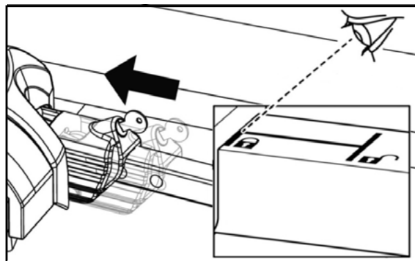
Figura 10: Blocco del dispositivo di fissaggio rapido
